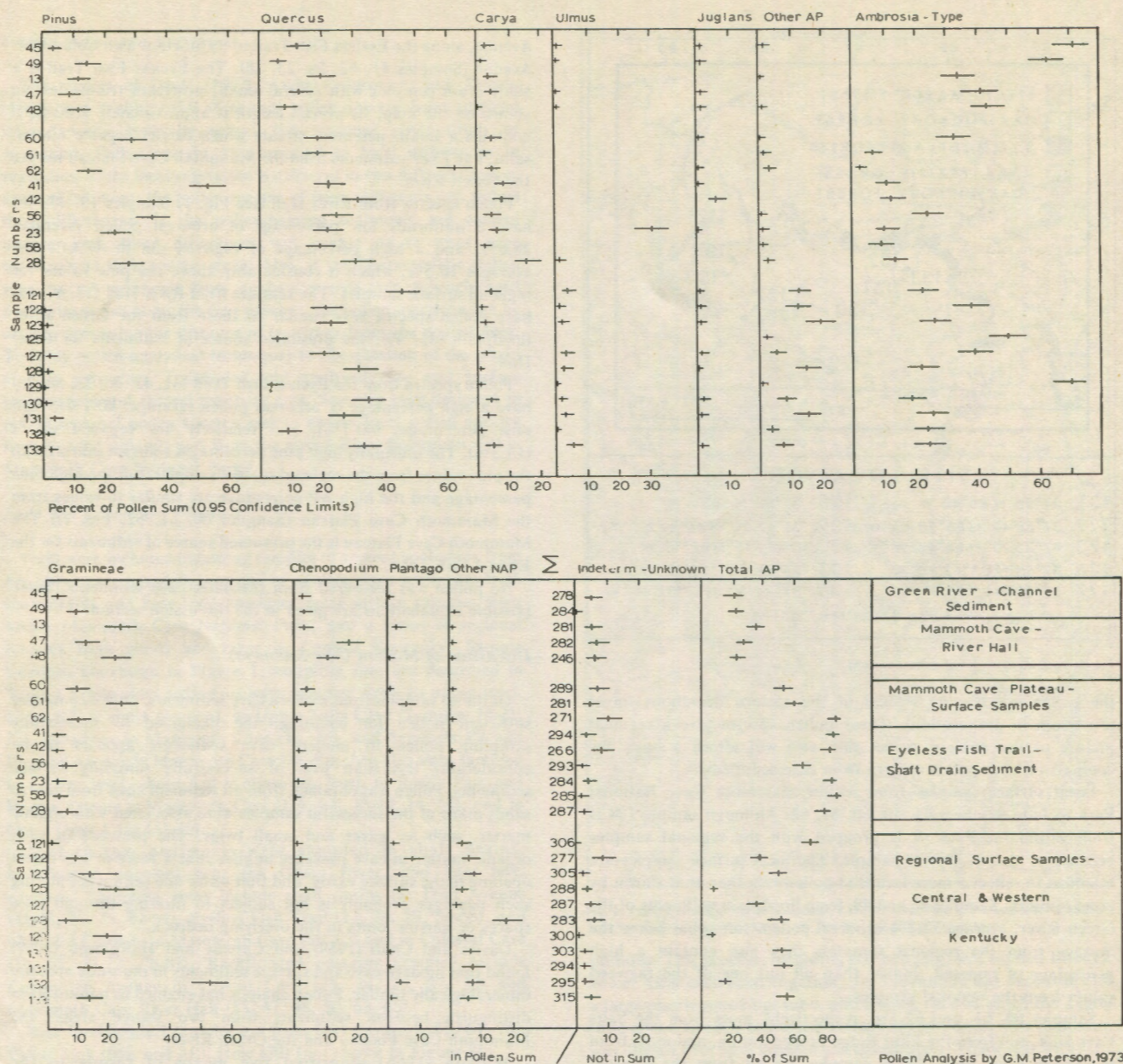
Fig. 3. Pollen spectra.
